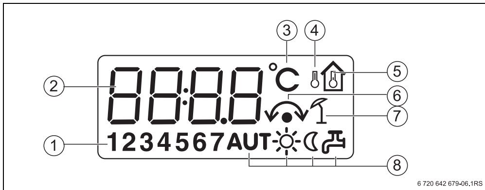
Рис. 6 Пояснення елементів дисплея
