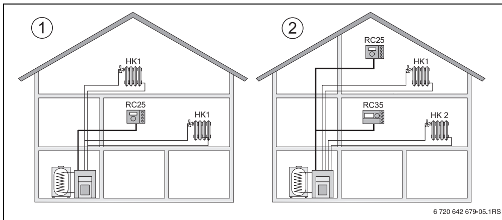
Рис. 2 Можливості для системи опалення з одним або двома контурами опалення
