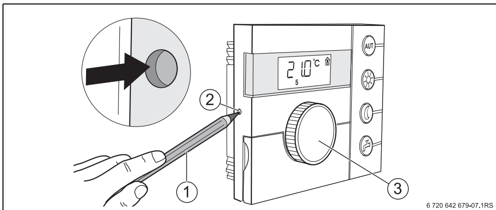
Рис. 7 Штифт-кнопка
